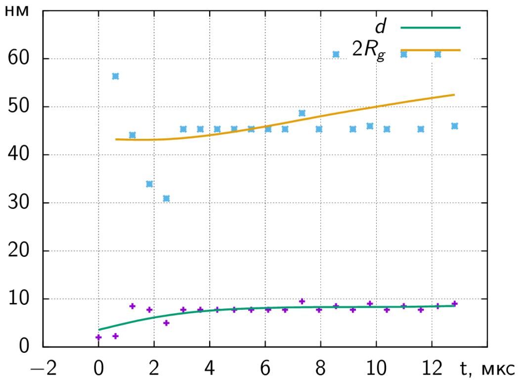
Рисунок 52 – Зависимости размера частиц ( d ) и кластеров ( 2R_g ) от времени при детонации заряда смеси тротила с гексогеном диаметром 30 мм.
