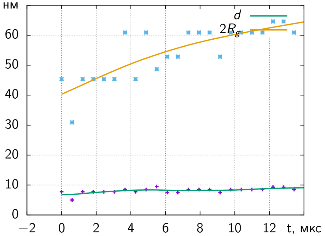
Рисунок 51 – Зависимости размера частиц ( d ) и кластеров ( 2R_g ) от времени при детонации заряда смеси тротила с гексогеном диаметром 20 мм.
